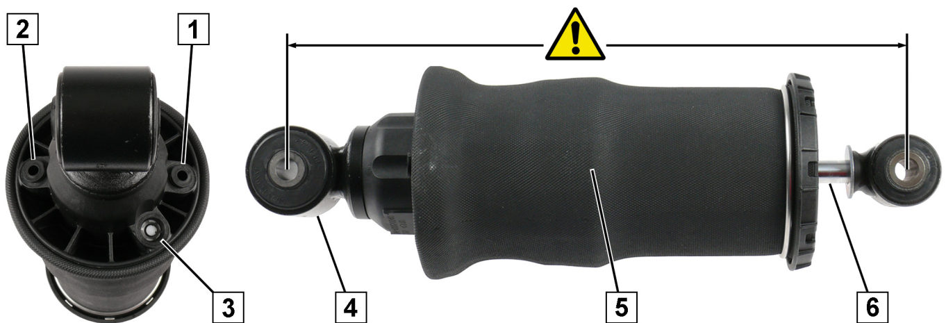
Fig. 1: CALM (Cabin Air Leveling Module) con 2 conexiones
